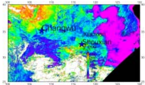
図 5 MOD09A1 データをモザイクし、緯度経度直交座標系に変換した画像例 ( 0.01^\circ )。
