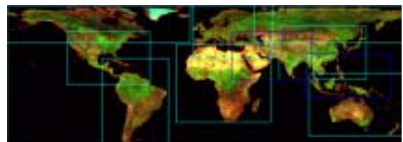
図3 SPOT VEGETATION で扱えるデータ範囲(画像中枠で示された地域)
