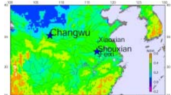
図2(b). 図2(a)と同様。ただし、 0.2^\circ 。データの抜けは見られなくなるが、海岸付近のデータが表現できない
