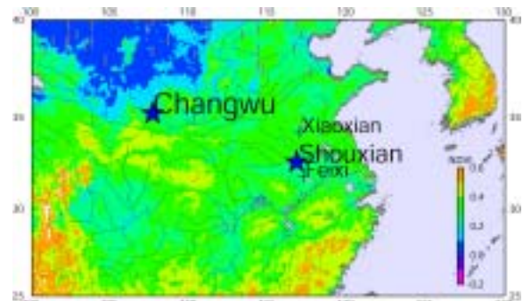
図2(a) PAL から緯度経度直交系座標( 0.1^\circ )に変換した画像。高緯度帯で見かけ上のデータの抜けが発生する
