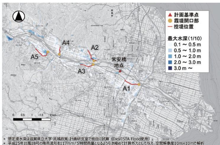
図4 安曇川氾濫域、霞堤位置と最大水深（10年確率）
