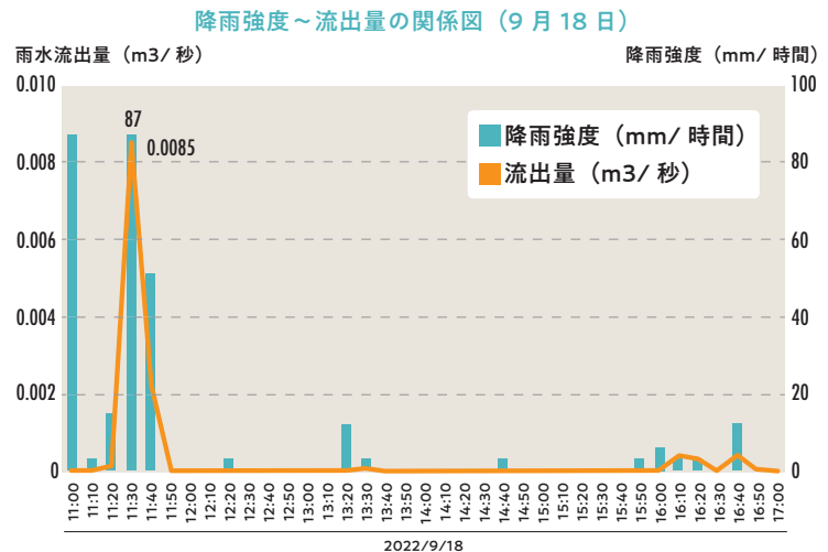
図 7 雨水流出量と降雨強度の関係図（2022年9/18,9/19,11/23計測）
