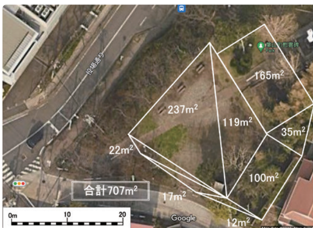
図6 三斜法による流出面積算定
