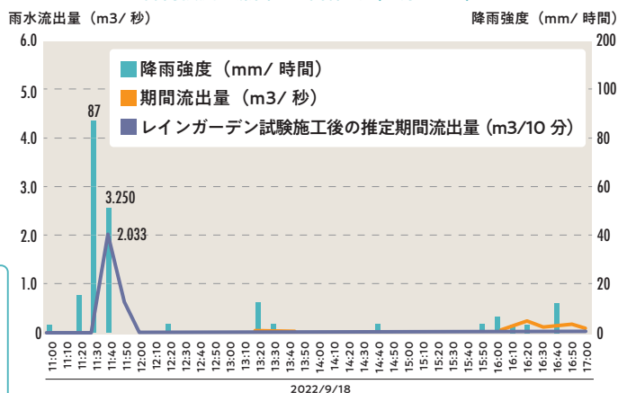
図12 レインガーデン試験施工適用前後の雨水流出量の試算結果 (2022年9月18日の測定結果に適用)
