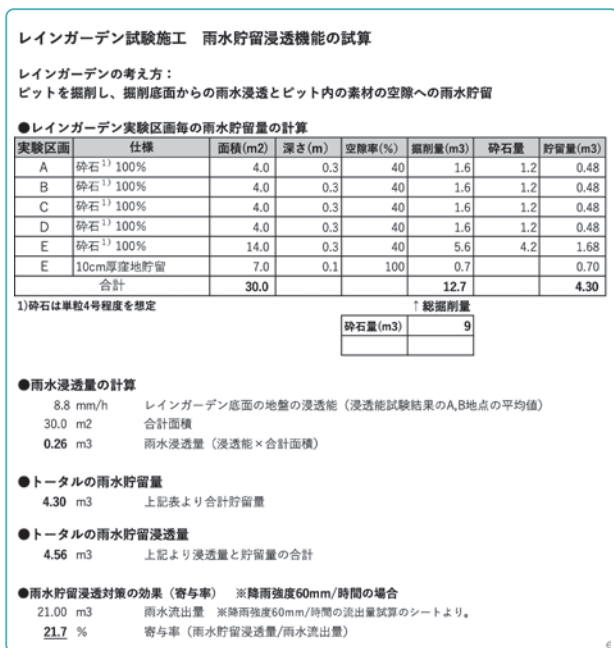
図11 レインガーデン試験施工諸元と雨水浸透貯留量の計算結果
