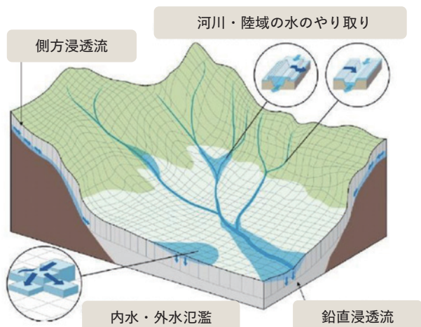
図 6 RRI モデルの概要
