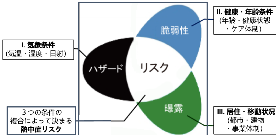
図2：3つの条件・状況（ハザード、脆弱性、暴露）によって決まる熱中症のリスクの模式図
