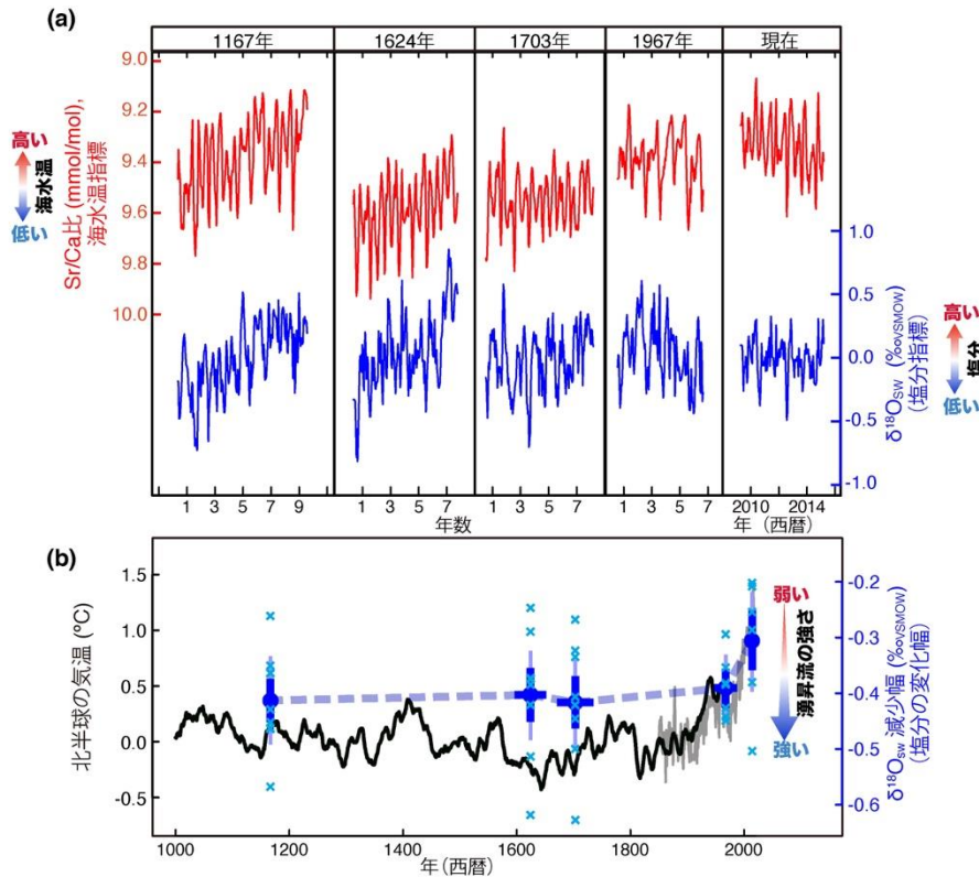
図 3. 復元した塩分変動から算出した塩分の減少幅と北半球の気温変化
