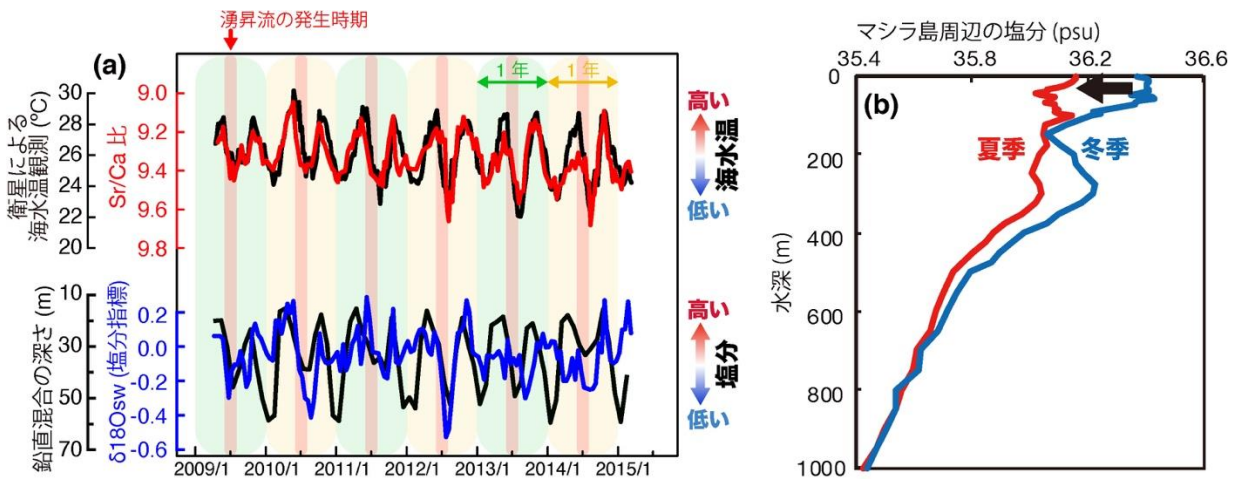
図 2. 現生サンゴから得られた記録とアラビア海マシラ島周辺の塩分の深度分布 (a) 上図は衛星による海水温観測記録（黒線）とサンゴ骨格に記録された Sr/Ca 比（赤線；海水温を反映）、 下図は鉛直混合の深さ（黒線；湧昇流のような深層と表層の海水循環を示す指標）とサンゴ骨格から 復元した海水の酸素安定同位体比（青線；塩分を反映）を示す。(b) 赤線と青線はそれぞれ夏季と冬 季の塩分の深度分布を示す。海洋表層では、冬季よりも夏季の塩分が低くなる（黒矢印）。水深 200m 程 度の深さにある低塩分の海水が夏季の湧昇流によって湧き上がるために、海洋表層の塩分が低下する。
