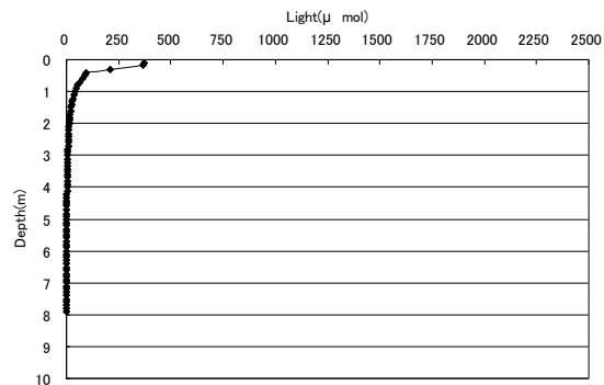
光量子 8/23 15時30分(地点5)
