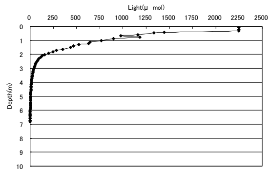
光量子 8/23 8時30分(地点5)
