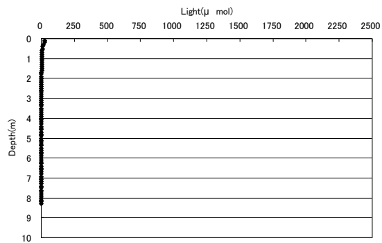
光量子 8/22 18時(地点1)
