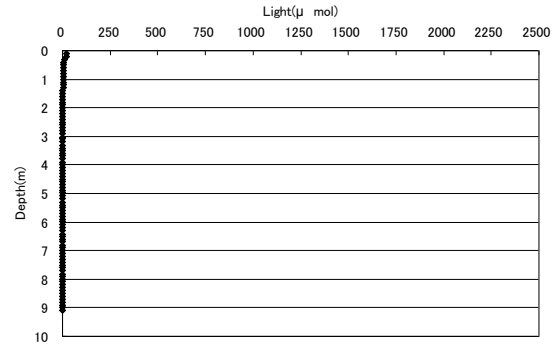
光量子 8/23 18時(地点2)
