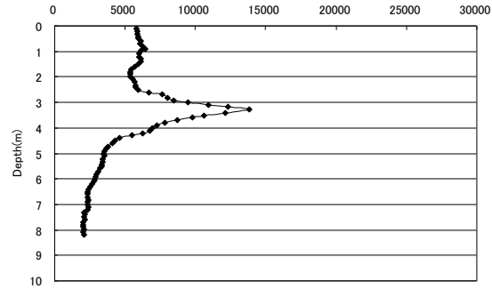
光量子 8/23 5時(地点1)
