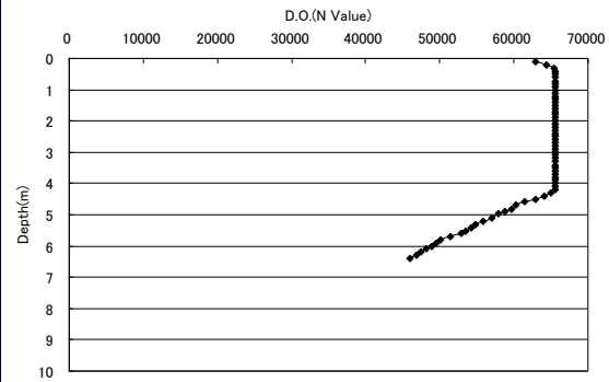
D.O. 8/22 11時30分(地点3)
