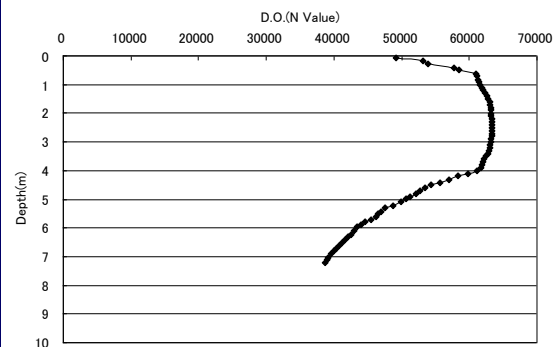
D.O. 8/23 15時30分(地点1)
