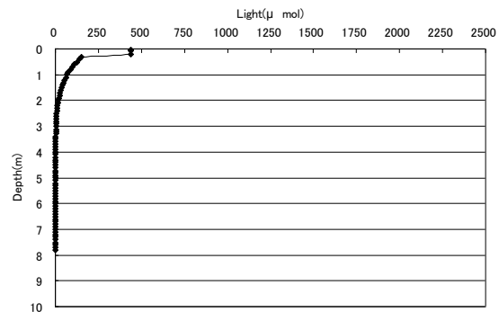
光子量 8/22 4時30分(地点3)
