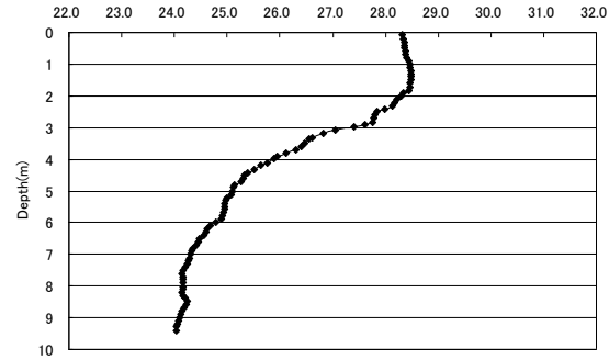
クロロフィル 8/23 5時(地点2)
