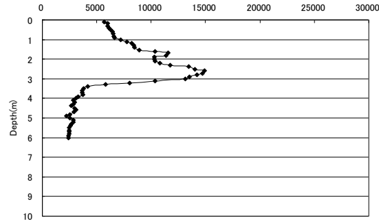
光量子 8/23 8時30分(地点4)
