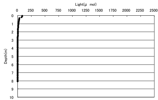
光量子 8/22 4時30分(地点1)
