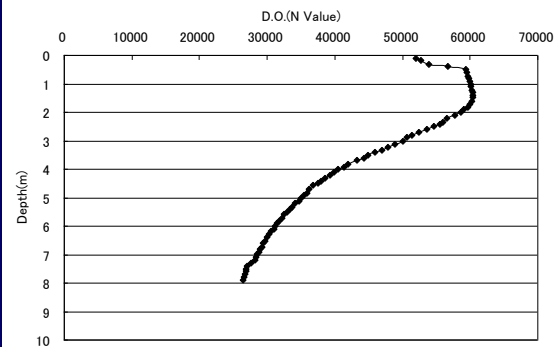
D.O. 8/23 15時30分(地点5)
