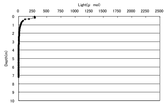
光量子 8/22 14時(地点1)
