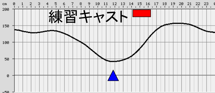
2006年08月22日 潮汐曲線 尼崎, AMAGASAKI
