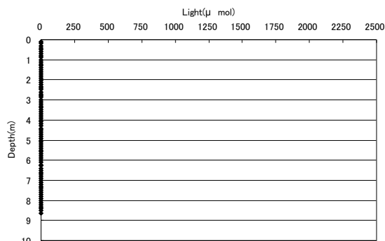
光量子 8/22 23時30分(地点2)
