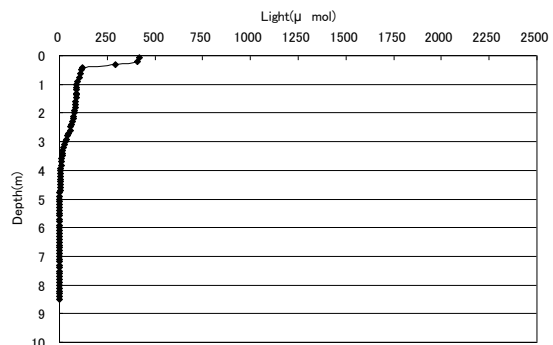
光量子 8/23 15時30分(地点2)
