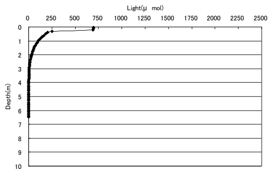
光量子 8/22 4時30分(地点4)
