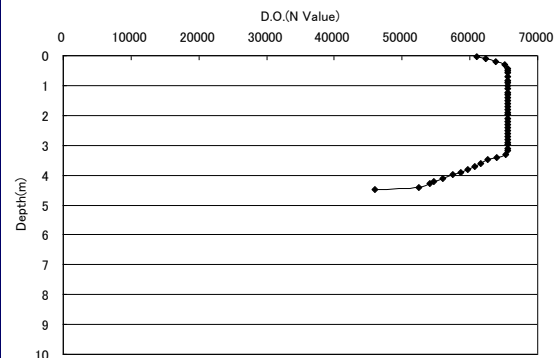
D.O. 8/22 8時(地点A)
