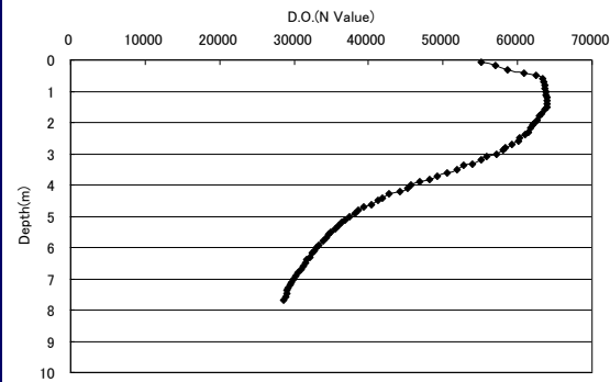
D.O. 8/23 8時30分(地点2)
