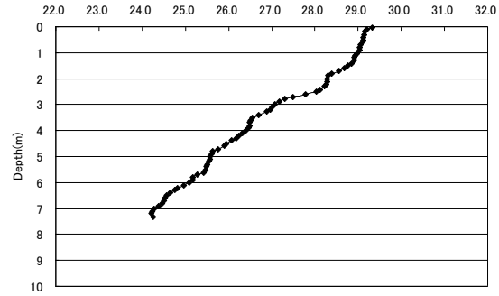
クロロフィル 8/22 8時(地点1)
