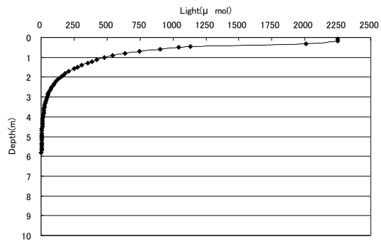
光量子 8/22 11時30分(地点1)
