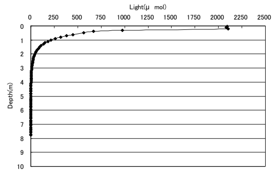
光量子 8/21 15時(地点1)
