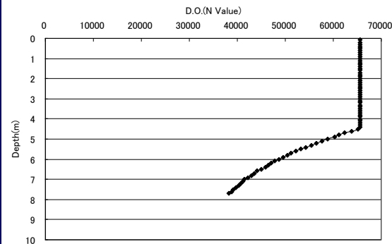
D.O. 8/22 11時30分(地点5)
