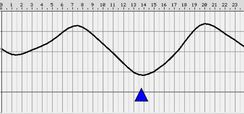
06年08月25日 潮汐曲線 尼崎, AMAGASAKI
