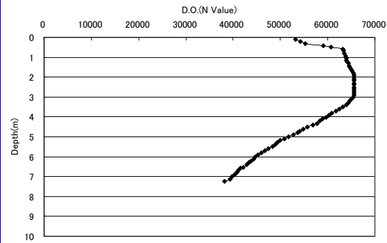
D.O. 8/23 15時30分(地点3)
