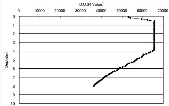
D.O. 8/22 23時30分(地点1)
