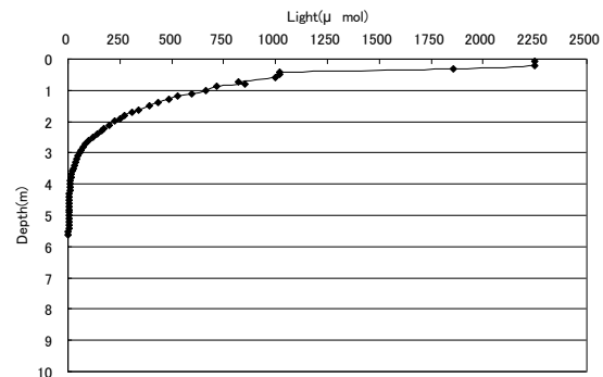
光量子 8/22 11時30分(地点4)
