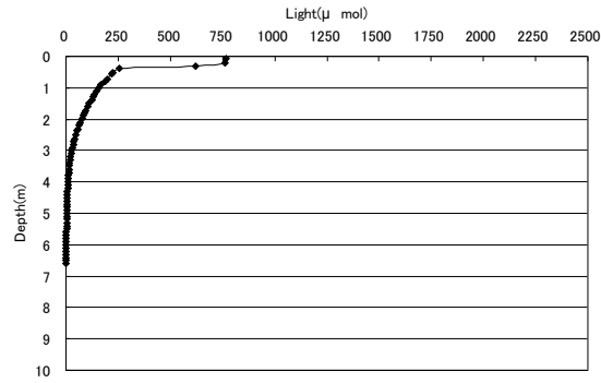
光量子 8/23 12時(地点3)
