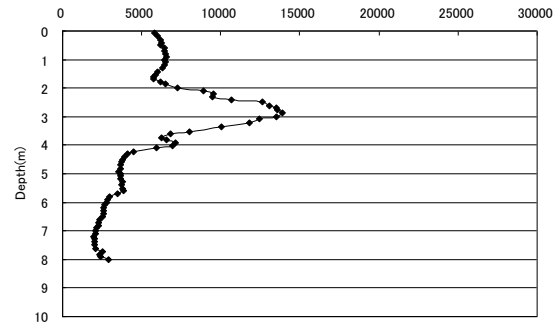
光量子 8/23 12時(地点2)
