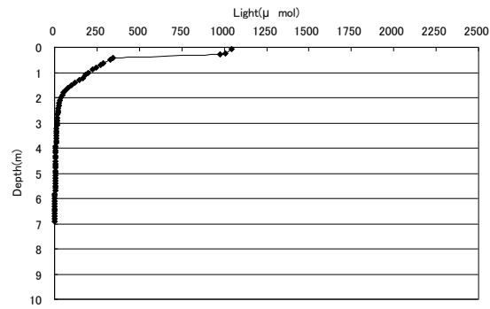
光量子 8/23 12時(地点5)
