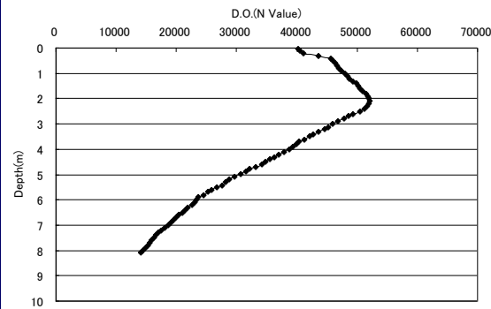
D.O. 8/22 4時30分(地点1)
