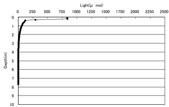
光量子 8/23 5時(地点3)
