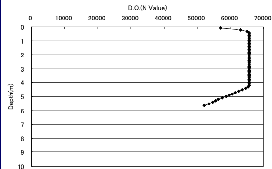
D.O. 8/22 11時30分(地点4)
