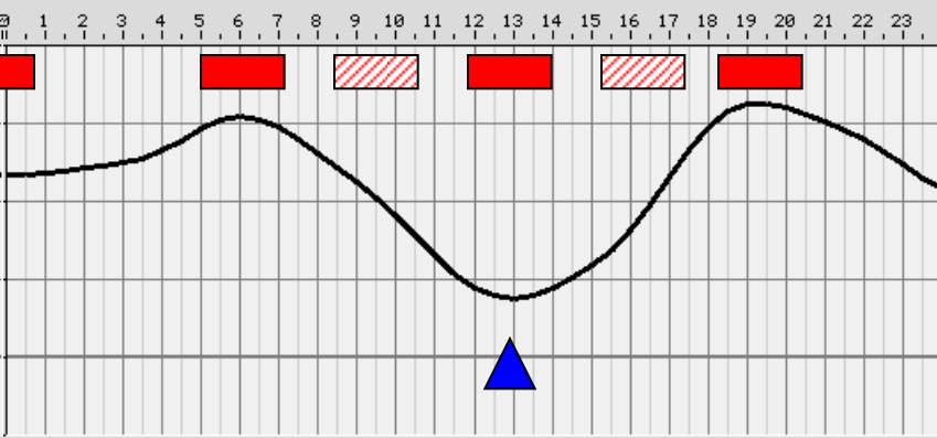
06年08月23日 潮汐曲線 尼崎, AMAGASAKI
