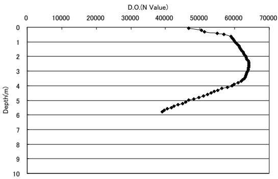
D.O. 8/22 23時30分(地点4)
