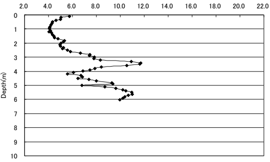
D.O. 8/23 8時30分(地点4)
