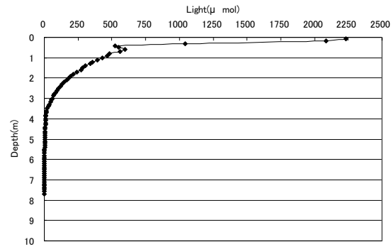
光量子 8/23 8時30分(地点2)
