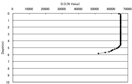
D.O. 8/22 11時30分(地点1)
