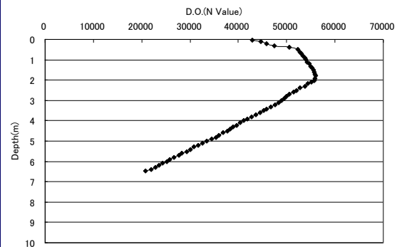
D.O. 8/22 4時30分(地点4)
