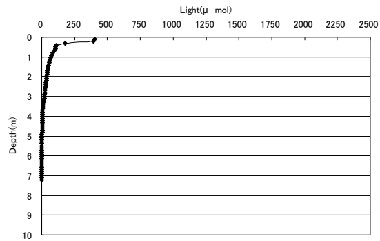
光量子 8/23 15時30分(地点3)
