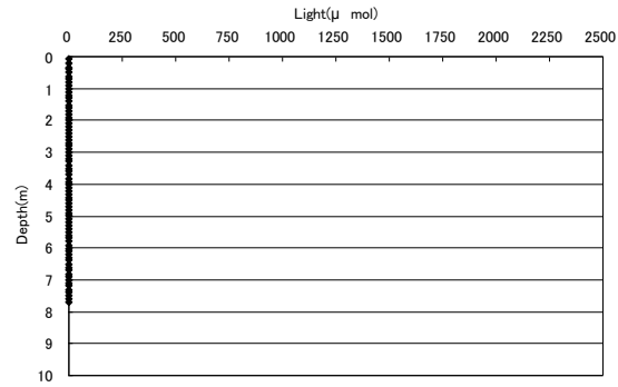
光量子 8/22 18時(地点3)
