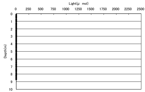
光量子 8/22 18時(地点5)
