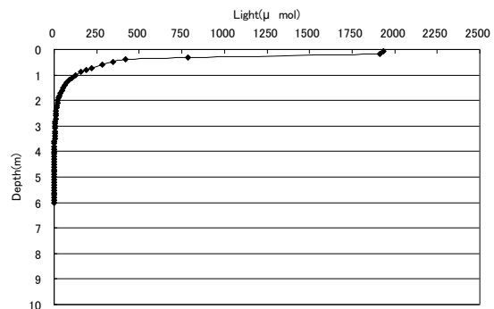
光量子 8/21 15時(地点4)
