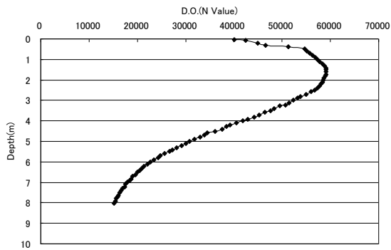
D.O. 8/22 4時30分(地点5)
