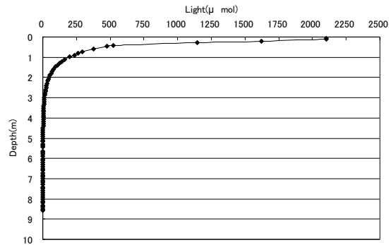
光量子 8/21 15時(地点2)
