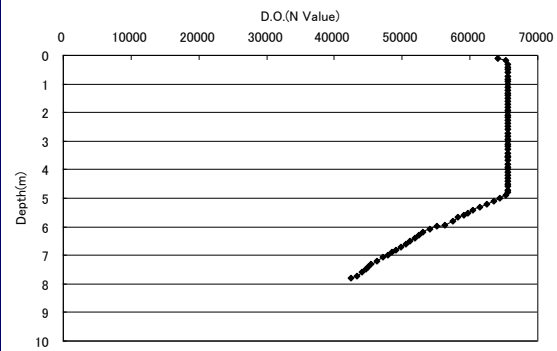
D.O. 8/22 11時30分(地点2)
